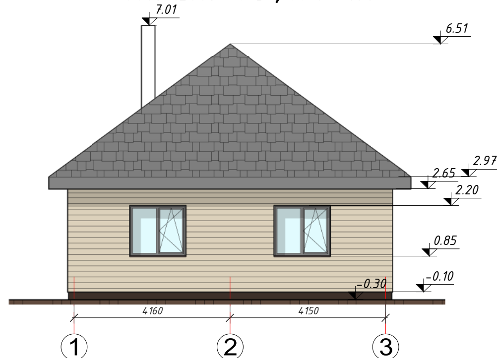
FASADAS "1-3", M 1 : 100
