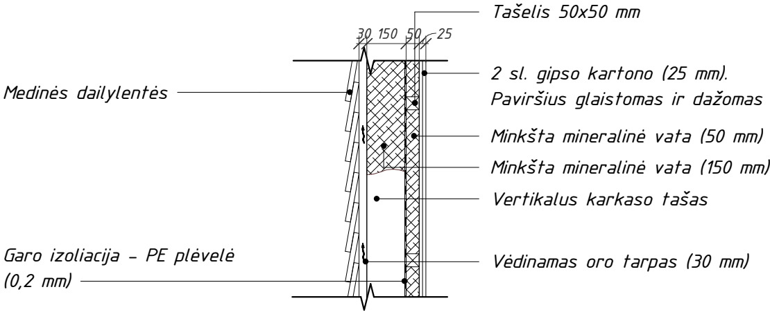
SN-1, M 1 : 20
