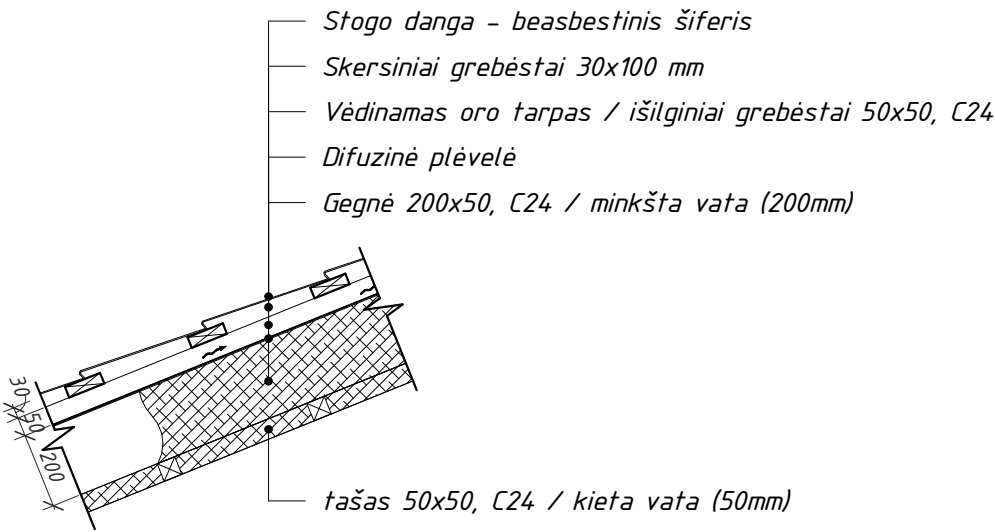
ST-1, M 1 : 20
