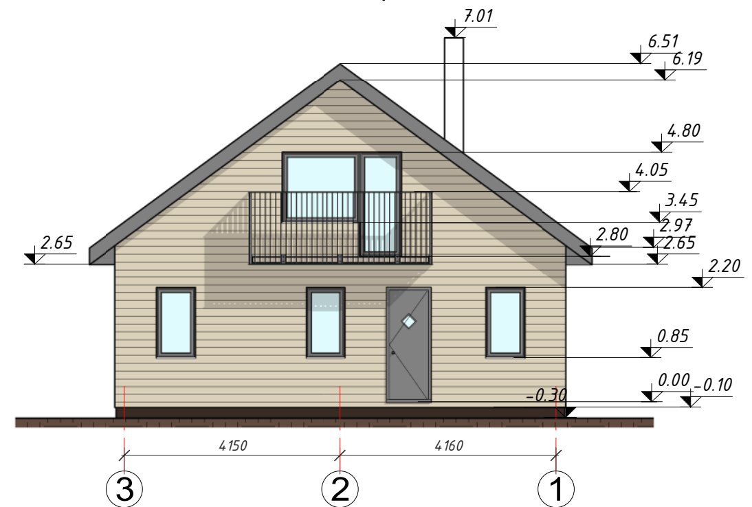
FASADAS "3-1", M 1 : 100
