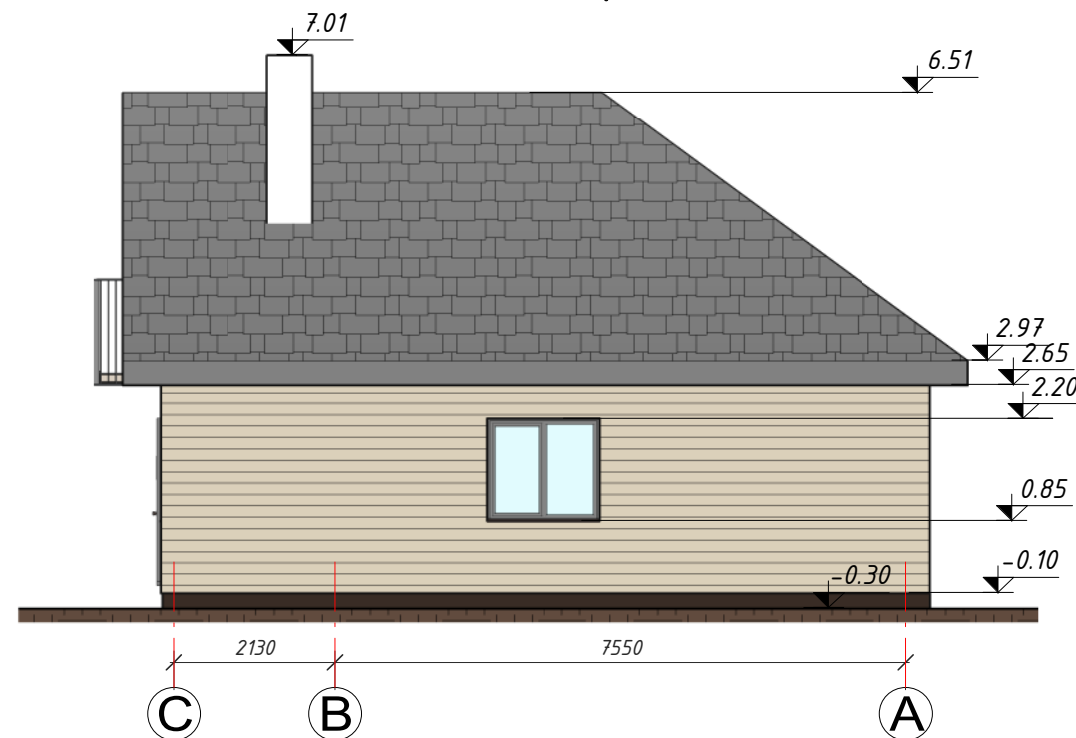
FASADAS "C-A", M 1 : 100
