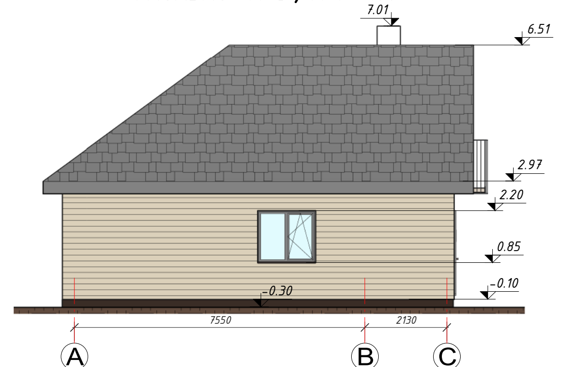
FASADAS "A-C", M 1 : 100
